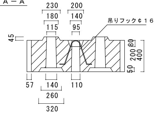
断面 A - A
