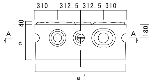
平面、底面図 350、500用
