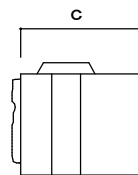
側面図 350、500用
