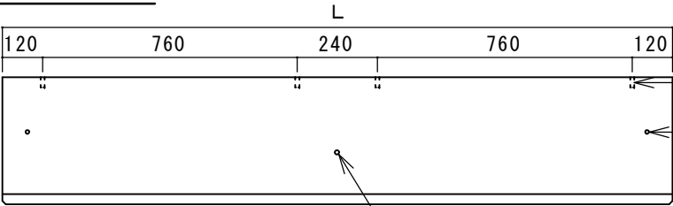
本体 側面図
