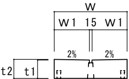
蓋 側面図
