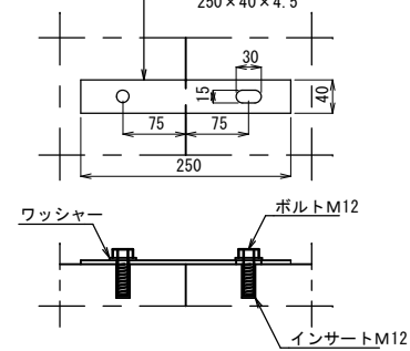
連結部詳細
