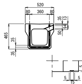
接続部詳細
