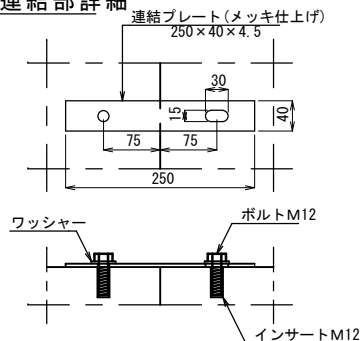
連結部詳細
